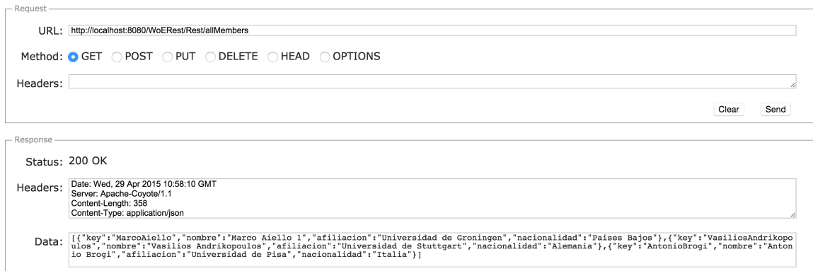
Figura 1.1.: Resultado de llamar al método allMembers del servicio Web.
