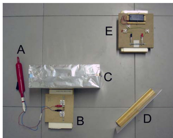
Figura 5. Reflexión: A, encendedor piezoeléctrico. B, emisor. C, caja recubierta de aluminio para proteger el detector de las ondas directas. D, espejo de aluminio. E, detector.
