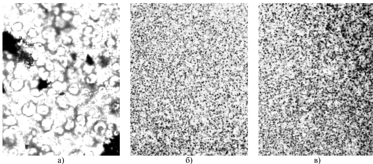
Рисунок 5 – Мікроструктура композиційного продукту в процесі його переробки в роторно-вихровому емульсорі: а) в початковий момент часу; б) після завершення механічної обробки при частоті обертання ротора 2000 об/хв; в) після завершення механічної обробки при частоті обертання ротора 3000 об/хв
