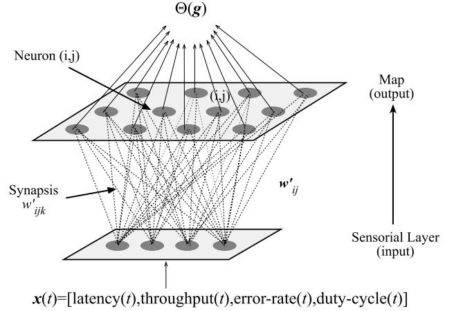
Fig. 2 SOM architecture
