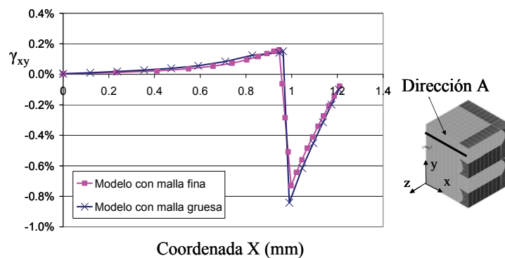
Fig. 11 - Evolución de las deformaciones de cortadura \gamma_{xy} a lo largo de la dirección A para los dos modelos considerados.
