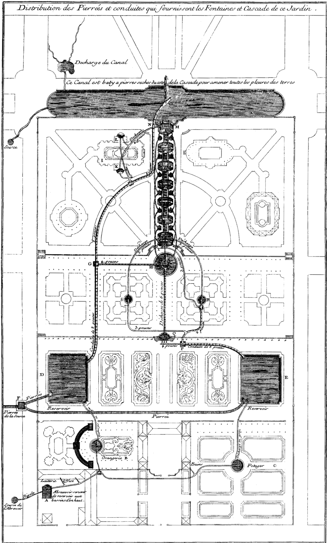
FIG. 69 Systeem voor watertoevoer (Dezallier 1747).
