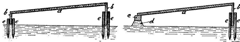
Fig. 65. Gewone kweekbakken Fig. 66. a = Raam. — b = plank van 30 cm. hoogte. — c = houten keper van 10 cm. breed. — d = dijkje met grond gevormd om de noodige hoogte te bekomen. — e = paaltjes om de plank recht te houden.
