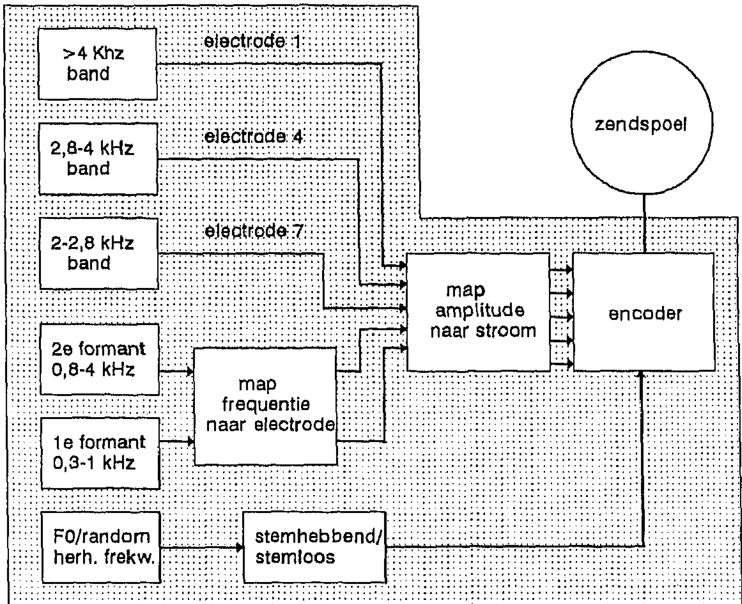
Fig. 3. Blokschema van het toegepaste 22-kanaals cochleair implantaat.
