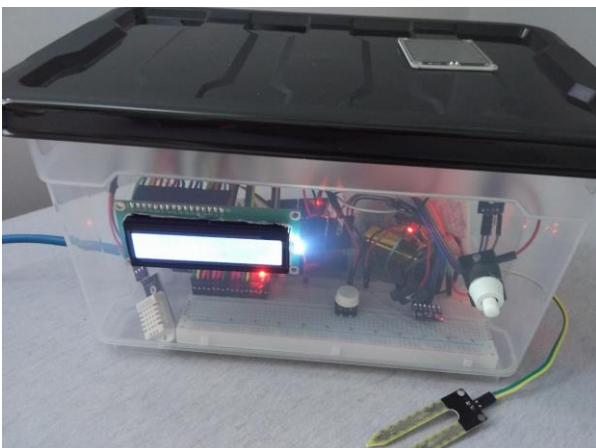
11. ábra Arduino alapú meteorológiai mérőszenzor
