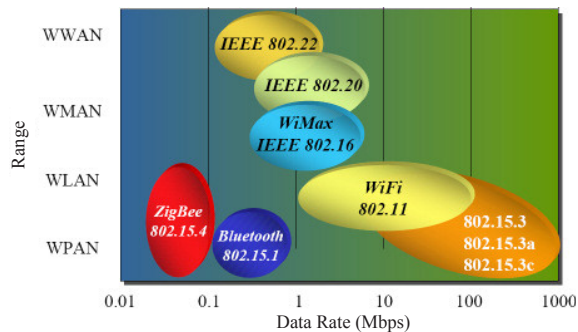
2. ábra: A ZigBee pozíciója
