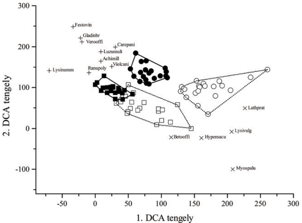
1. ábra. A mintaterületek 2004-es prezencia-abszencia adatokon alapuló DCA-ordinációja. (● déli gyepek kaszált kvadrátok, ○ déli gyepek kontroll kvadrátok; ■ északi gyepek kaszált kvadrátok, □ északi gyepek kontroll kvadrátok, + A kaszált területeken gyakoribb fajok, × a kontroll területeken gyakoribb fajok. A növényfajok esetében 8 betűs rövidítéseket használtunk: Achimill = Achillea millefolium , Betooffi = Betonica officinalis , Carepani = Carex panicea , Gladinbr = Gladiolus imbricatus , Holclana = Holcus lanatus , Hypemacu = Hypericum maculatum , Lathprat = Lathyrus pratensis , Lysinumm = Lysimachia nummularia , Lysivulg = Lysimachia vulgaris , Myospalu = Myosotis palustris , Ranupoly = Ranunculus polyanthemos , Verooffi = Veronica officinalis , Violcani = Viola canina .)
