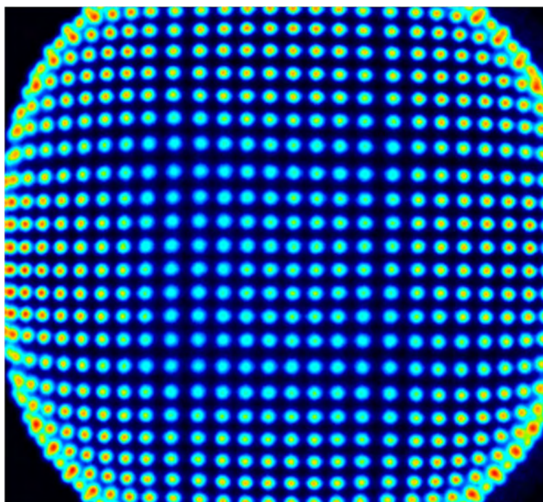
Σχήμα 4.18. Πρωτογενής εικόνα διακριτοποιημένου σπινθηριστή CsI(Tl) με κυψελίδες 3 \times 3 \times 5 \text{ mm}^3
