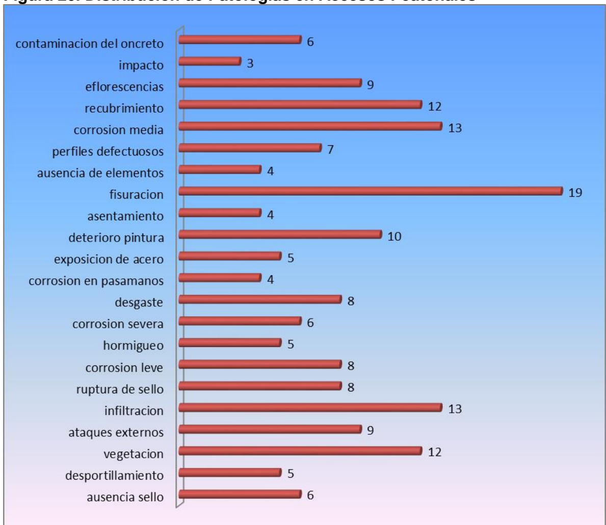
Figura 20. Distribución de Patologías en Accesos Peatonales
