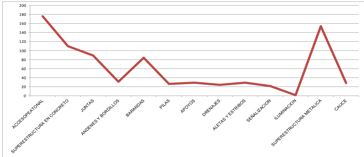
Figura 18. Categorización de Daños Totales por Elementos que Componen los puentes
