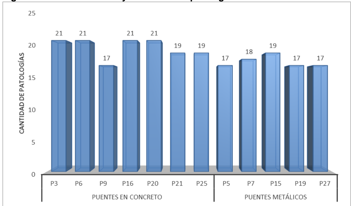
Figura 21. Puentes con mayor número de patologías
