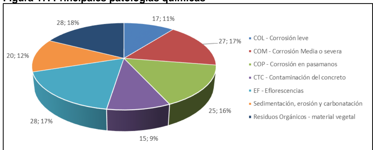
Figura 17. Principales patologías químicas
