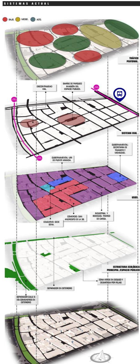
Figura 10: Estructuras urbanas.
