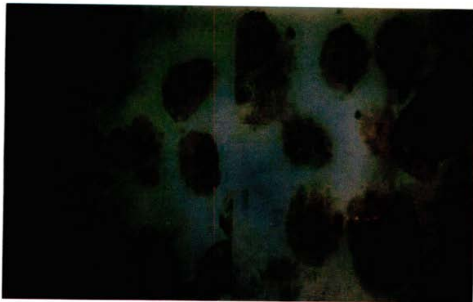
شکل ۲: تعداد هستک‌ها در سلول دیپلوئید ( 2n ) و سلول تتراپلوئید ماهی قزل‌آلای رنگین کمان ( 4n ) (بزرگنمایی \times 100 )
