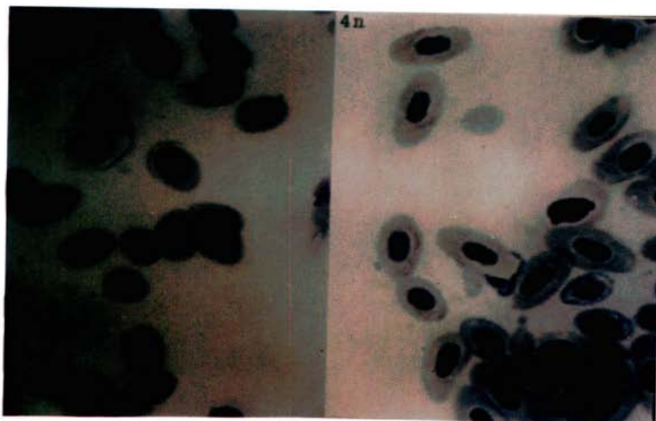
شکل ۱: مقایسه گلبول قرمز دیپلوئید ( 2n ) و گلبول قرمز تتراپلوئید ( 4n ) ماهی قزل‌آلای رنگین کمان (بزرگنمایی \times 100 )
