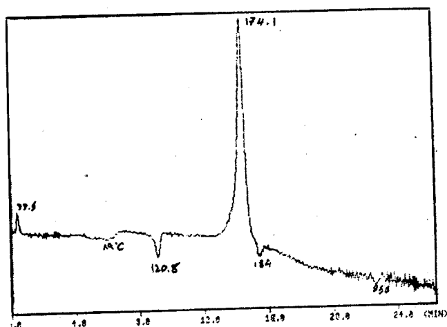
نمودار ۸: طیف DSC مستر بیج (زرد پر رنگ) حاوی عامل پفزا
