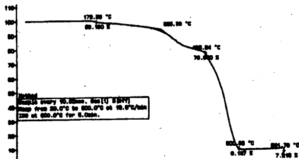
نمودار ۵: طیف TG مستر بیچ (زرد کم رنگ) حاوی عامل شبکه کننده
