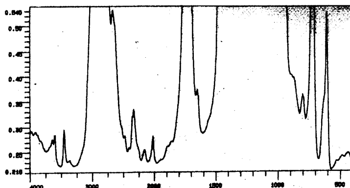
نمودار ۲: طیف FTIR فیلم کوپلیمر اتیلن- وینیل استات مجهول با ضخامت ۰/۲۳۴ میلی متر
