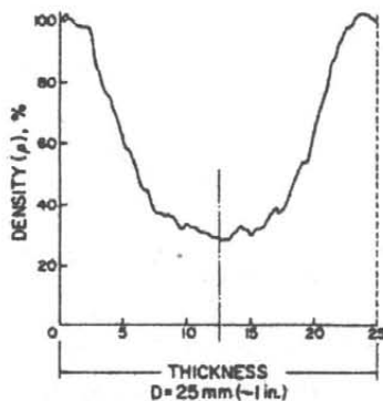
شکل ۳: پروفیل وزن مخصوص یک اسفنج ساختمانی ترکیبات اصلی بکار رفته در اسفنجهای ساختمانی معمولاً عبارتند از:
