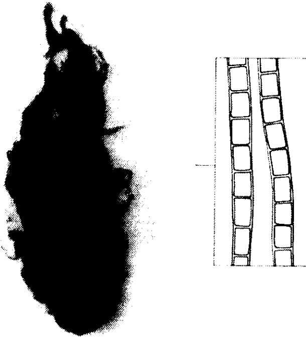
شکل ۲: نمونه‌ای جلبک سبز Rhizocolonium implexum
