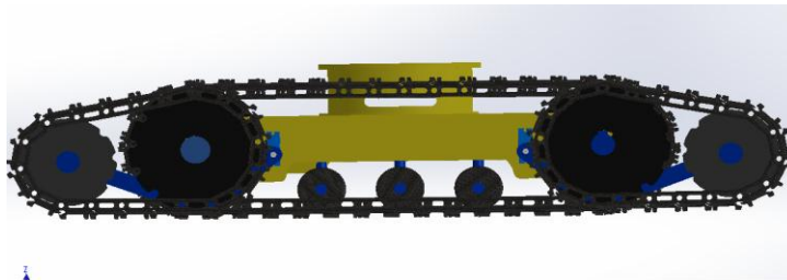
Figura 27. Suspensión
