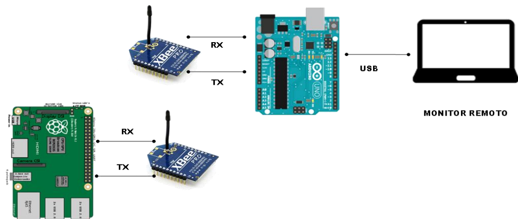
Figura 15. Conexiones sistema de comunicación
