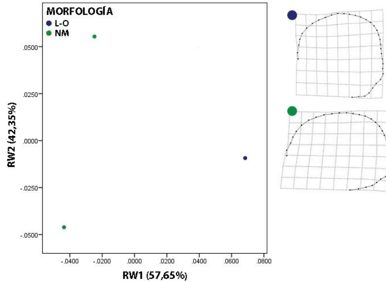
Figura 5.5. Análisis de Relative Warps y grillas de deformación asociadas a los agrupamientos morfológicos de la muestra PS. L-O: lámbdico-occipital; NM: no modificado.
