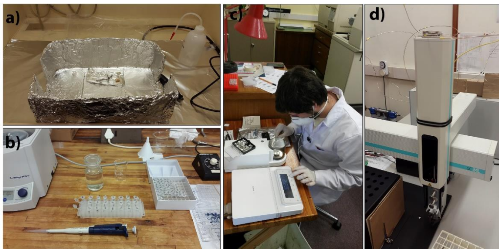
Figura 4.7. Pre-tratamiento de la muestra e instrumental para el análisis de \delta^{18}\text{O} sobre esmalte. a) Área para la remoción del esmalte; b) Área de añadido de reactivos y centrifugado; c) Micro-pesado de polvo de esmalte; d) Inyector de helio.
