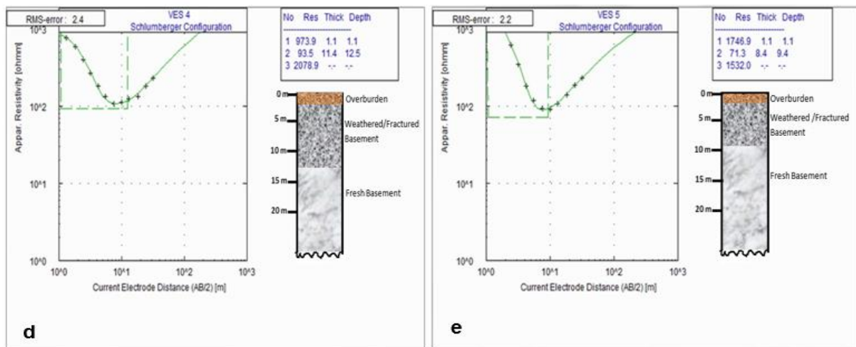
Fig. 4: VES curves and geoelectrical parameters for (d) VES 4 and (e) VES 5.
