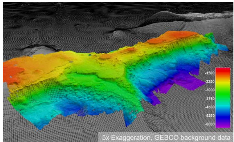
Dreidimensionale Darstellung des Suiko Vulkans basierend auf bathymetrischen Datensätzen, die während SO264 erstellt wurden.
