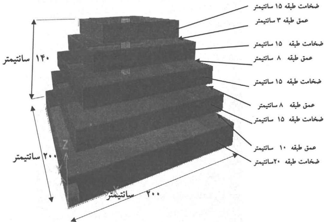
شکل ۵: سازه ابداعی زیستگاه مصنوعی دریایی شاه میگو
