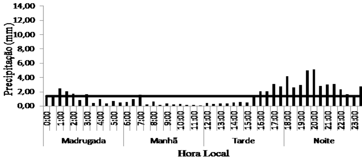
Figura 7. Variabilidade média horária da precipitação durante o período menos chuvoso (1999 a 2011) na Floresta Nacional de Caxiuanã, Melgaço/PA.
