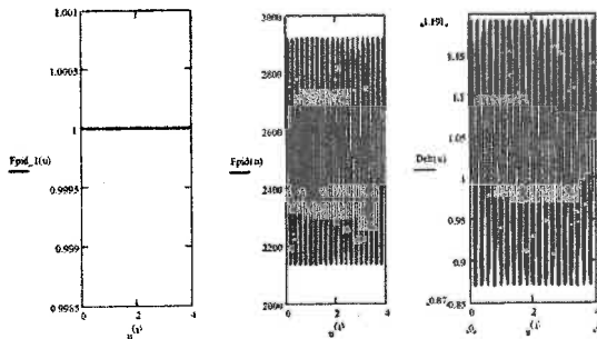
Рис.1. Моменти в часі t = u^{(1)} роботи Fpid\_1(u) = 1 і прослаблення Fpid\_1(u) = 0 підвісу; пружні сили Fpid(u)H , які діють у ньому, та зміна коефіцієнта k_{дин\ перес} = \Delta del(u) динамічного перевантаження ланок гідрокрана з моменту підхоплення вантажу із жорсткої опори
