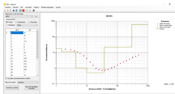
Figura 1. Vista de la ventana principal del programa SEVs. A la izquierda se observa el panel de introducción de datos y a la derecha el panel con el gráfico de salida.
