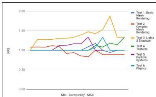
Figura 4. Comparación de resultados en diferentes calidades de renderizado.
