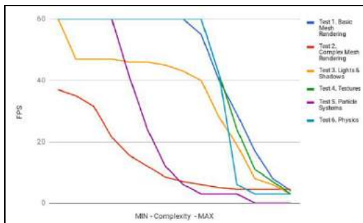
Figura 3. Evolución de los cuadros por segundo (FPS, sigla en inglés) en cada prueba.
