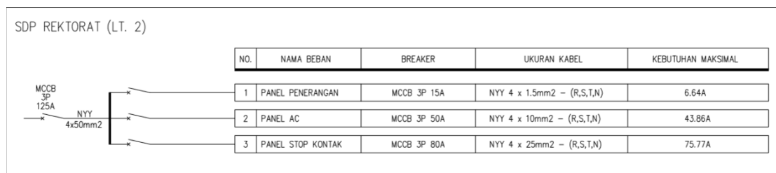
Gambar 9. SDP Rektorat Lantai 2
