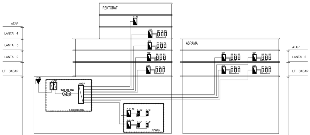
Gambar 2. Skematik
