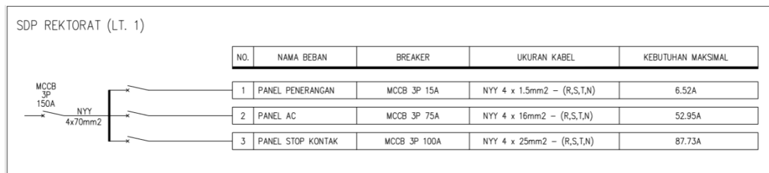
Gambar 8. SDP Rektorat Lantai 1
