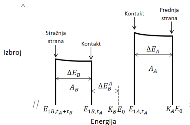
Slika 3.12: Energijski spektar dvoslojnog tankog filma [1].
