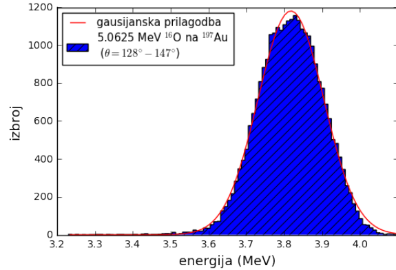
Slika 5.8: Energijski spektar za raspršenje ^{16}\text{O}^{3+} energije 5.0625 MeV na 10 nm ^{197}\text{Au} na mjerenom rasponu kutova.
