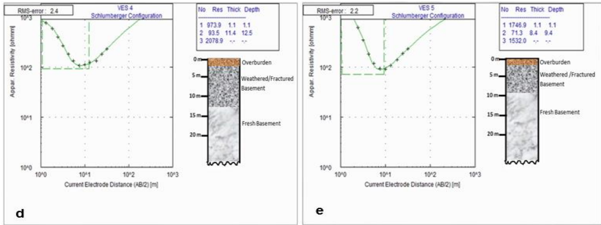
Figure 4 VES curves and geoelectrical parameters for (d) VES 4 and (e) VES 5.
