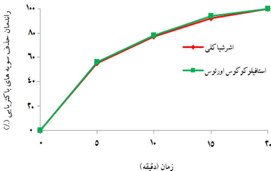
نمودار شماره ۳: تأثیر زمان تماس بر روی راندمان فرآیند الکترولیز
