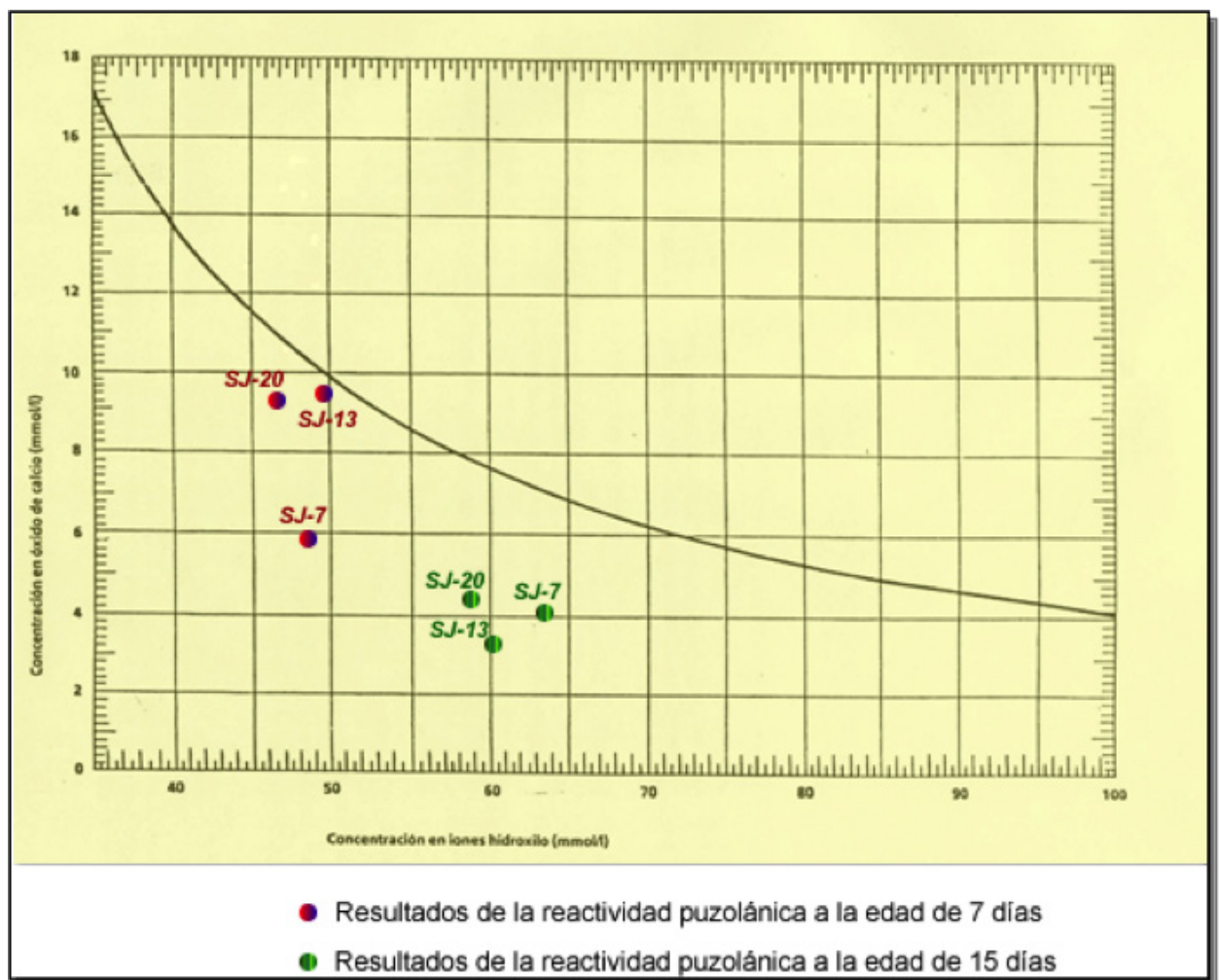
Figura 86. Representación gráfica de la reactividad puzolánica de algunas muestras de zeolita del yacimiento San José - Los Escullos, Cabo de Gata , en disolución saturada en \text{Ca}(\text{OH})_2 , para períodos de 7 y 15 días, respectivamente (Fuente: Costafreda, J.L., 2008).
