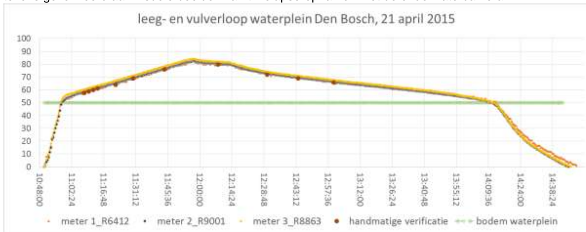
Afbeelding 3. Vul- en leegloopgedrag van het waterplein, vastgelegd door 3 waterstandsmeters geverifieerd met handmatige metingen (stippen)
