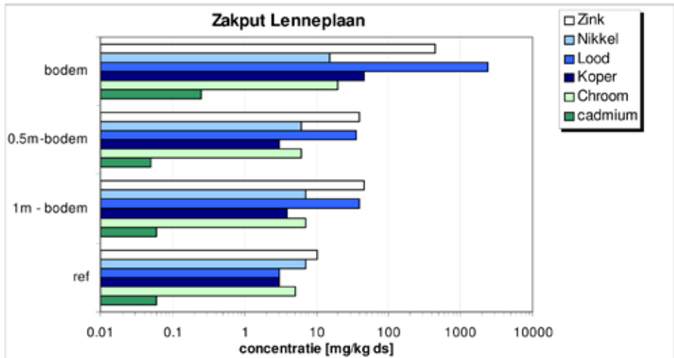
Figuur 7: Concentraties onder de bodem van een infiltratievoorziening [Tauw, 1999].
