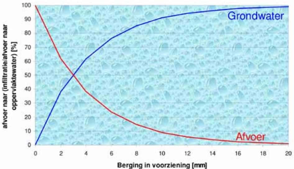
Figuur 3: Relatie tussen berging en overstort bij een doorlatendheid van n ( kd=3 m/d) [PAO cursus wateropgave 2011].
