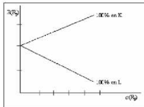
Figura 13. Índice de correlación \rho = -1 .
