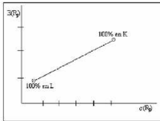
Figura 12. Índice de correlación \rho=1 .
