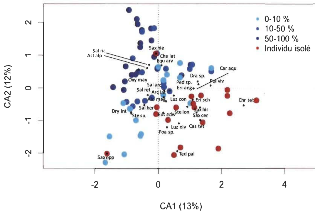
Figure C.2 Représentation des deux premiers axes d'une ordination (CA) illustrant la distribution de 74 parcelles suivant un gradient d'abondance de Salix richardsonii en fonction des communautés végétales associées. Les classes d'abondance de S. richardsonii sont représentées par des points de différentes couleurs et les espèces par les trois premières lettres du genre et de l'espèces.
