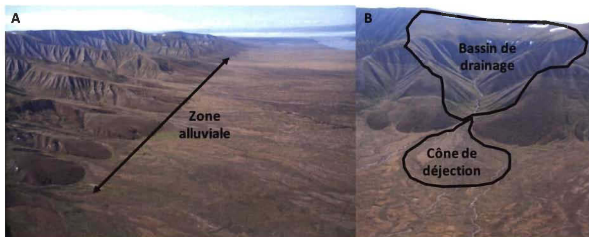
Figure 1.6 (A) Photo de la zone colluviale/alluviale à la base des versants sud de la vallée Qarlikturvik et (B) Photo d'un cône alluvial et de son bassin de drainage typique de la vallée Qarlikturvik.
