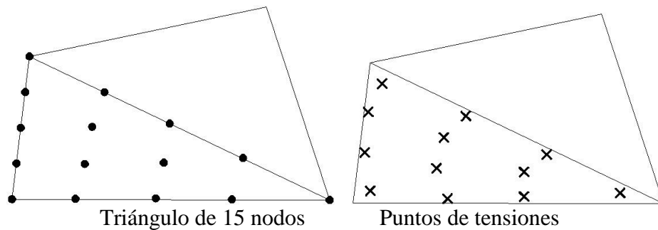
Figura 5. Esquema de elemento tipo de 15 nodos (Plaxis VB, 2004)
