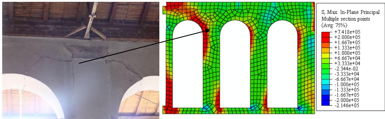
Figura 10. Simulación de daños en arcos de mampostería
