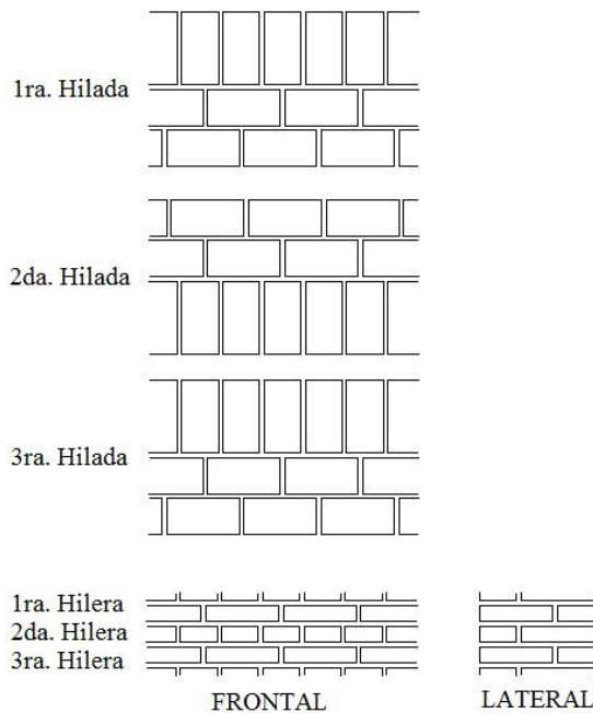
c) Aparejos para los muros de mampostería de 0,75 m (mampuesto de cabeza y dos de soga)
