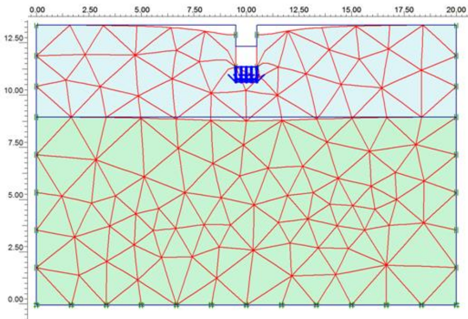
Malla deformada Desplazamiento máximo: 20\text{E}^{-3}\text{m} Desplazamiento amplificado 50 veces
