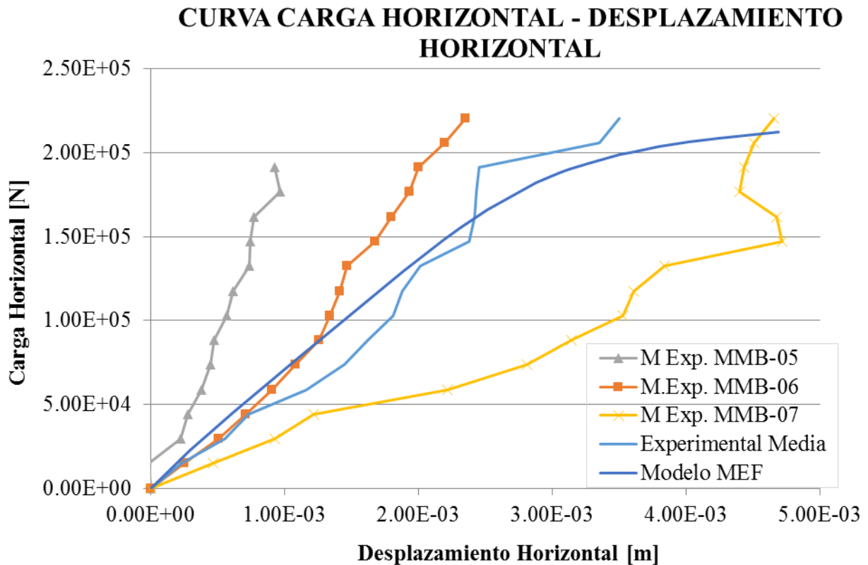
Figura 4. Simulación en cargas horizontales.
