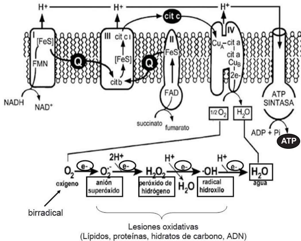
Figura 1. Transporte mitocondrial como generador de ERO.
