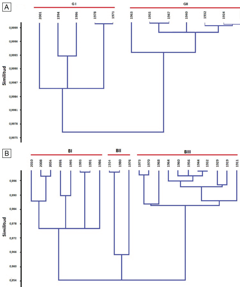
Figura 3. Cluster jerárquico según algoritmo UPGMA ( paired group ) e índice de similitud Morisita. A) Para el testigo GeoB 13813-4 se utilizaron las variables: relación Ca/Ti y la media aritmética del tamaño de grano. Se obtuvieron dos grupos, GI y GII; B) En el testigo BAR1 las variables utilizadas fueron: fracciones granulométricas (arena, limo y arcilla) y la tasa de sedimentación. Se obtuvieron tres agrupaciones, BI, BII y BIII. Los grupos se indican con líneas rojas. Figure 3. Hierarchical clustering using the UPGMA ( paired group ) algorithm and Morisita similarity index. A) For core GeoB 13813-4 the ratio Ca/Ti and the arithmetic mean of grain size were used and two groups were distinguished (GI and GII); B) for core BAR1, the percentages of sand, silt, clay and sedimentation rate were used, and three groups were identified (BI, BII and BIII). The red lines indicate those groups.
