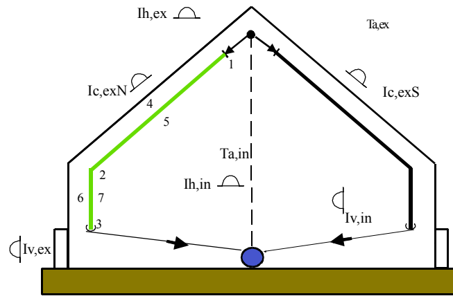
Figura 1. Esquema del invernadero de vidrio con las bolsas plásticas y la ubicación de los sensores
