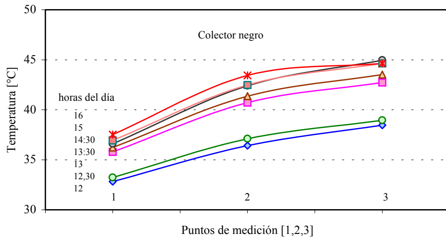
Figura 8. Variación de la temperatura del agua a lo largo de las bolsas transparentes
