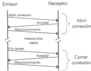
Figura 6: Pasos en una conexión TCP.
