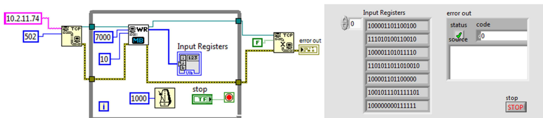
Figura 10: Sub-vi de prueba para la toma de datos vía Modbus TCP en labVIEW.
