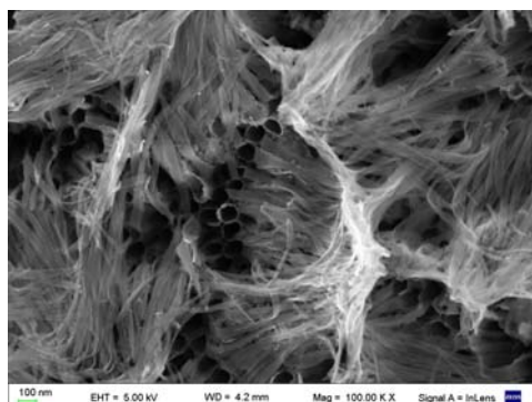
(d) LN-V50-TTL
