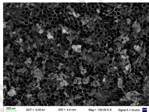
(b) LN-V30-TTL
