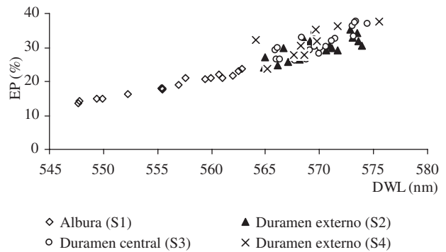
Figura 4. Albura, duramen externo (S2, S4) y duramen central (S3) representados en el espacio colorimétrico por sus coordenadas “x” e “y” y por su longitud de onda dominante (DWL) y pureza de excitación (EP).
