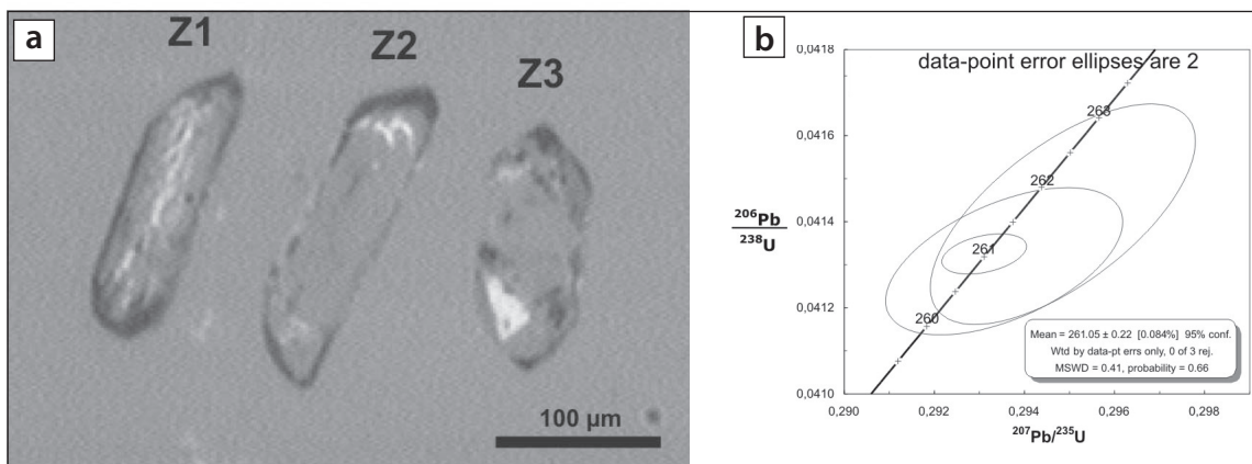
Figura 5: Muestra YK-442: a) Microfotografía de los circones datados de una muestra de afloramiento del cerro Colón (muestra CC03); b) Diagrama de concordia de los circones de la muestra YK-442. Los errores están informados a 2-σ.
