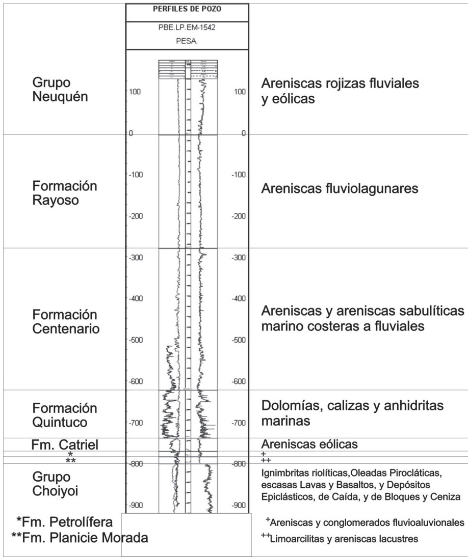
Figura 3: Columna estratigráfica simplificada del borde noreste de la cuenca Neuquina.
