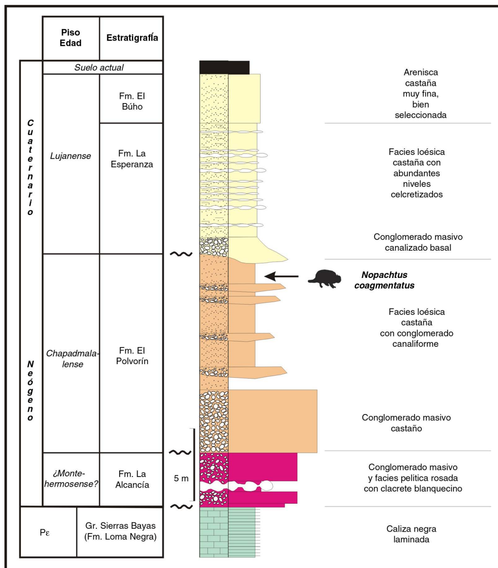
Fig. 2.—Perfil geológico de la Cantera Alcantara.
