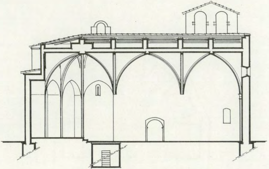
Secció longitudinal.
