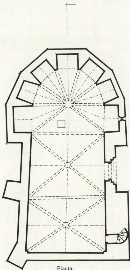
Planta.
