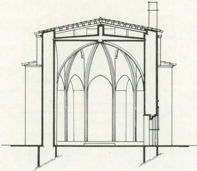
Secció transversal.
