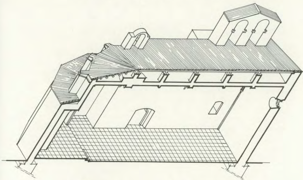
Secció isomètrica.
