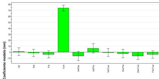
Figura 3. Coeficientes del modelo lineal mostrando el efecto de los parámetros investigados en el diámetro de las nanofibras (Con: concentración, Vol: voltaje, Dis: distancia al colector, Flo: Caudal).
