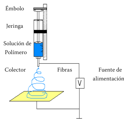
Figura 1. Esquema de una máquina de electrohilatura.
