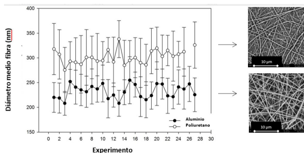
Figura 6. Diámetro medio de las nanofibras de gelatina recogidas sobre un colector de aluminio (conductor) y otro de poliuretano (no conductor) para diferentes condiciones de operación (voltaje, distancia al colector y caudal) y para soluciones de 80 mg/ml en HIPF
