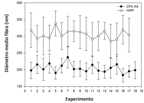
Figura 4. Diámetro medio de las nanofibras de gelatina obtenidas para diferentes condiciones de operación (voltaje, distancia al colector y caudal) y para soluciones preparadas con dos disolventes diferentes (80 mg/ml en HIPF y 300 mg/ml en ácido acético (AA) al 25 % v/v)
