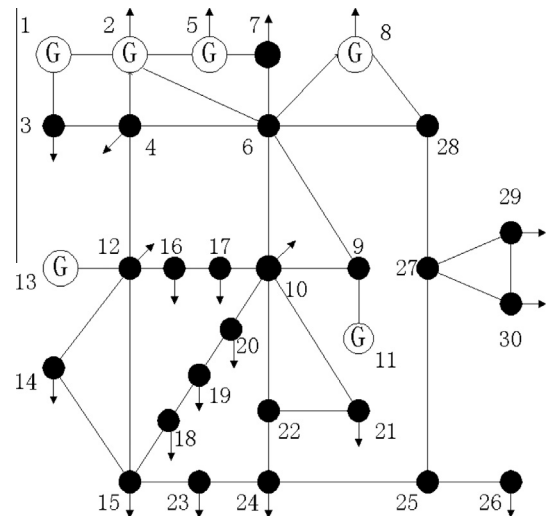
Fig. 6. IEEE 30-bus test system.
