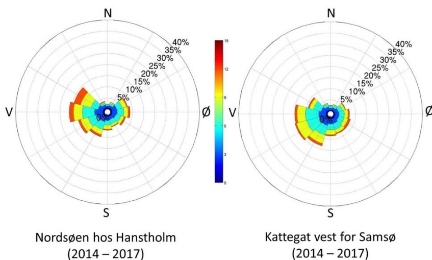
Figur 6.7.2. Vindroser med angivelse af frekvens (%) af vindretning. Vindroserne er beregnet på baggrund af vind-data (hver sjette time) fra CMEMS for perioden 2014-2017. Farveskala viser vindhastighed i m/s.
