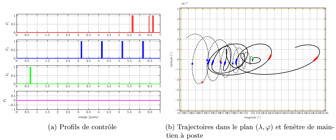
FIGURE 3.23 — — : solution du problème 3.8 (équivalence en effet) avec \zeta_c = [0.95 \ 0.9 \ 0.95 \ 0.95] , - - : solution du problème 3.11 d’optimisation des instants de commutation pour lequel les contraintes de maintien à poste sont prises en compte au moyen d’une fonction de pénalisation.
