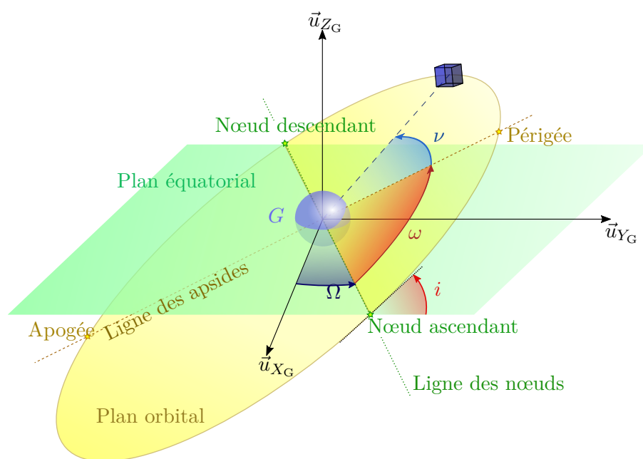
FIGURE 1.1 – Illustrations des éléments orbitaux classiques
