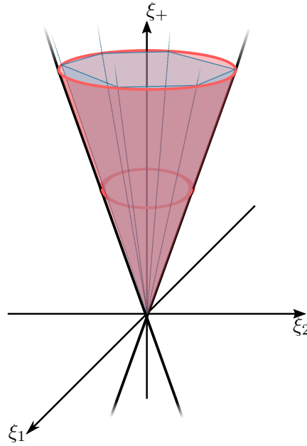
FIGURE K.2 – Ensembles \mathcal{C}^{+0} (rouge) et \mathcal{C}_{K_{xy}^+}^{+0} (bleu).
