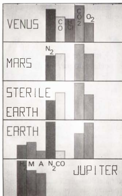
Taula 2. Composició de les diferents atmòsferes dels planetes (segons dibuix original de Jim Lovelock).
