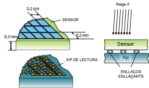
Figura 3: Esquema d'un detector de píxels
